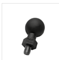
Kugelelement mit M8-Gewinde Ersatzteil für Universalhalter Ball joint with M8-thread Spare part for universal holder EKT-091 M8 Gewinde / Thread
