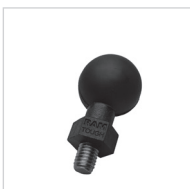
Kugelelement mit M8-Gewinde Ersatzteil für Universalh. 1, 2, 3 Ball joint with M8-thread Spare part for universal h. 1,2,3 EKT-091 M8 Gewinde / Thread
